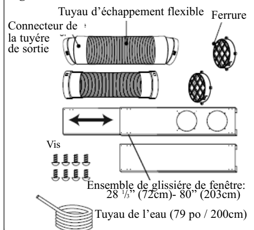
Fig. 1 ACCESSOIRES D'INSTALLATION
